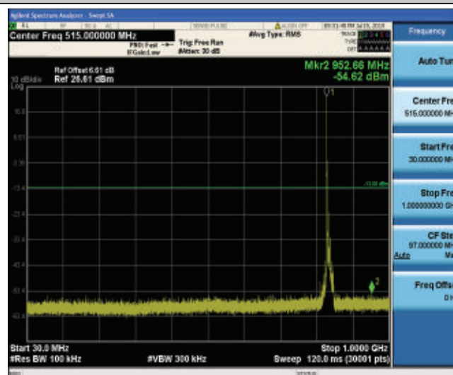
Band26 10MHz QPSK 26915 1RB#0
