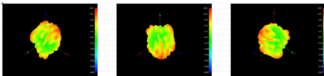
5850MHZ
