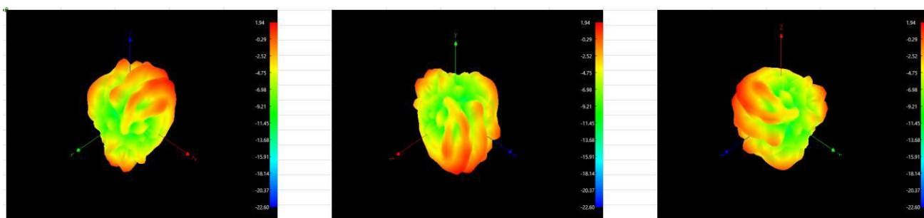
5500MHZ
