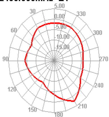
2450.000MHz E1
