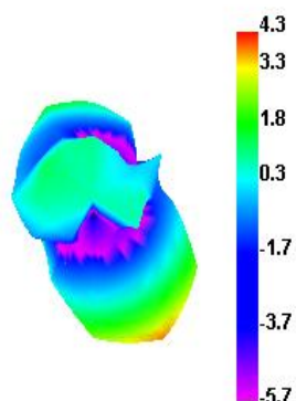
2450.000MHz E1
