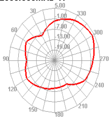
2500.000MHz H
