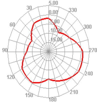
2400.000MHz E2
