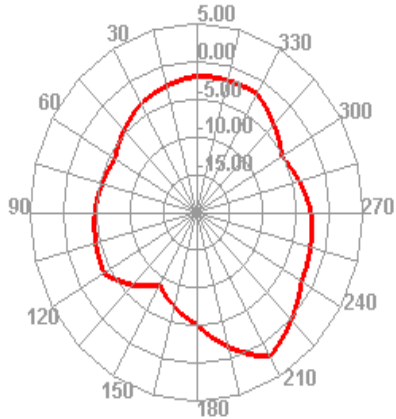
2400.000MHz E1
