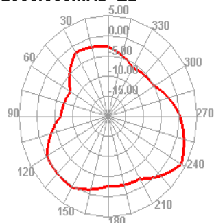
2500.000MHz E2
