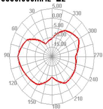
5550.000MHz E2
