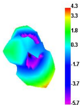
2500.000MHz
