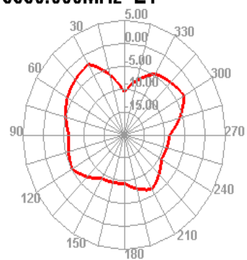
5550.000MHz E1
