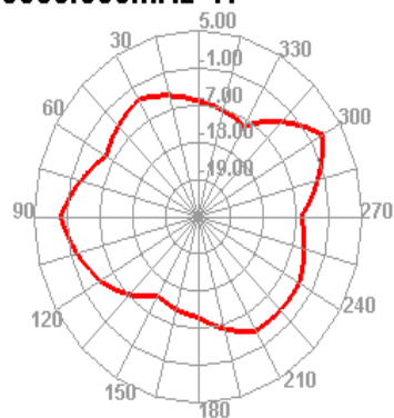
5550.000MHz H
