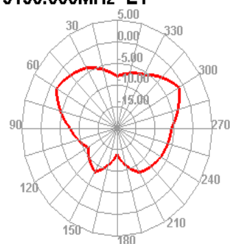
5150.000MHz E1
