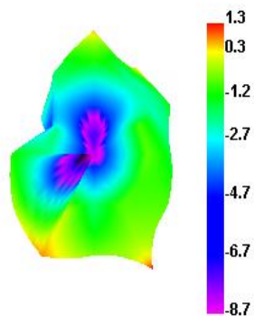
5550.000MHz
