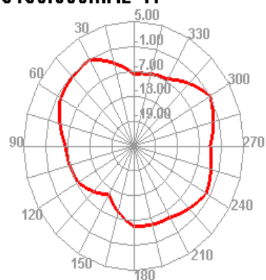
5150.000MHz H
