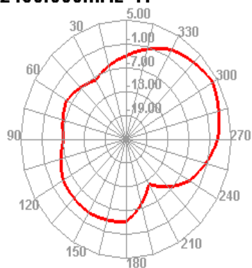
2450.000MHz H
