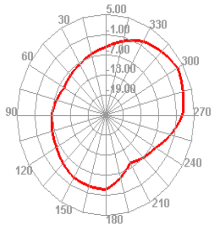
2400.000MHz H
