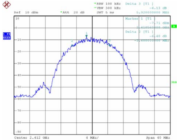
802.11b 2412MHz
