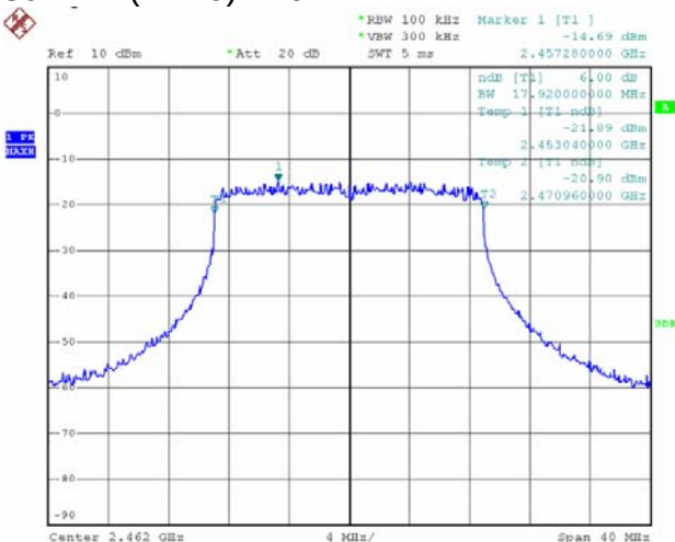
802.11n(HT20) 2462MHz
