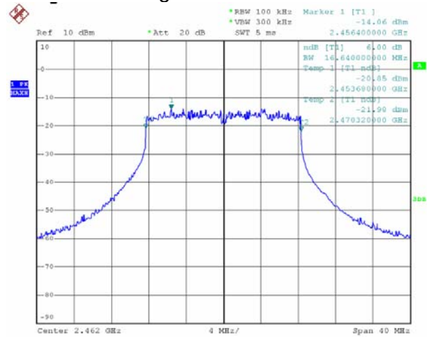
802.11g 2462MHz
