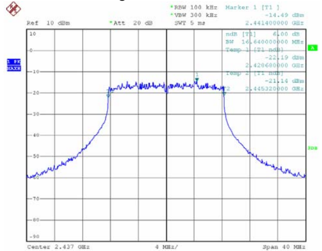
802.11g 2437MHz
