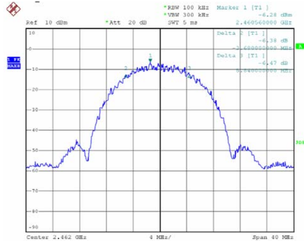
802.11b 2462MHz
