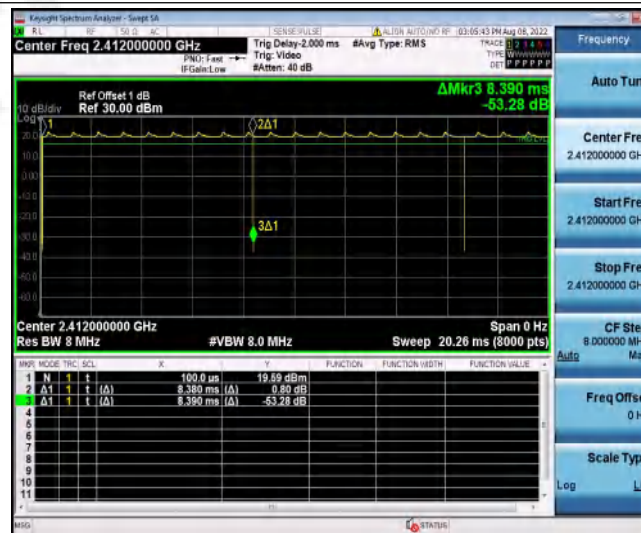
11B_Ant1_2412
