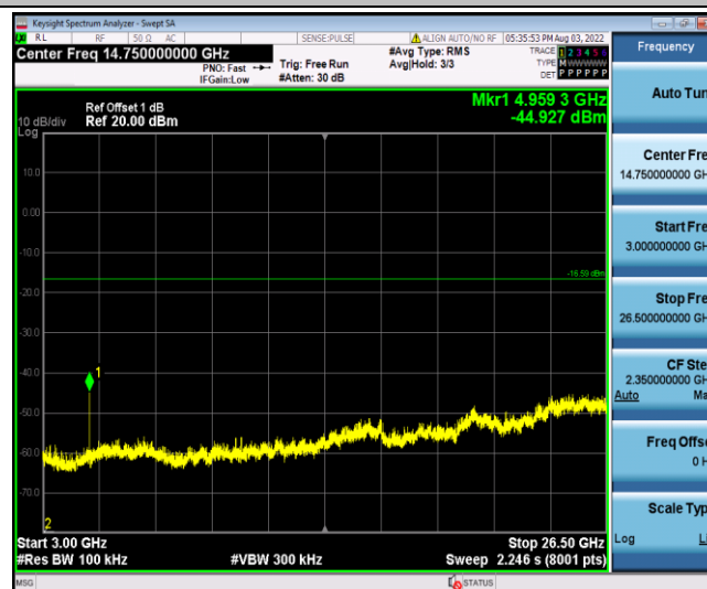
BLE_BT4.0_Ant2_2480_3000~26500
