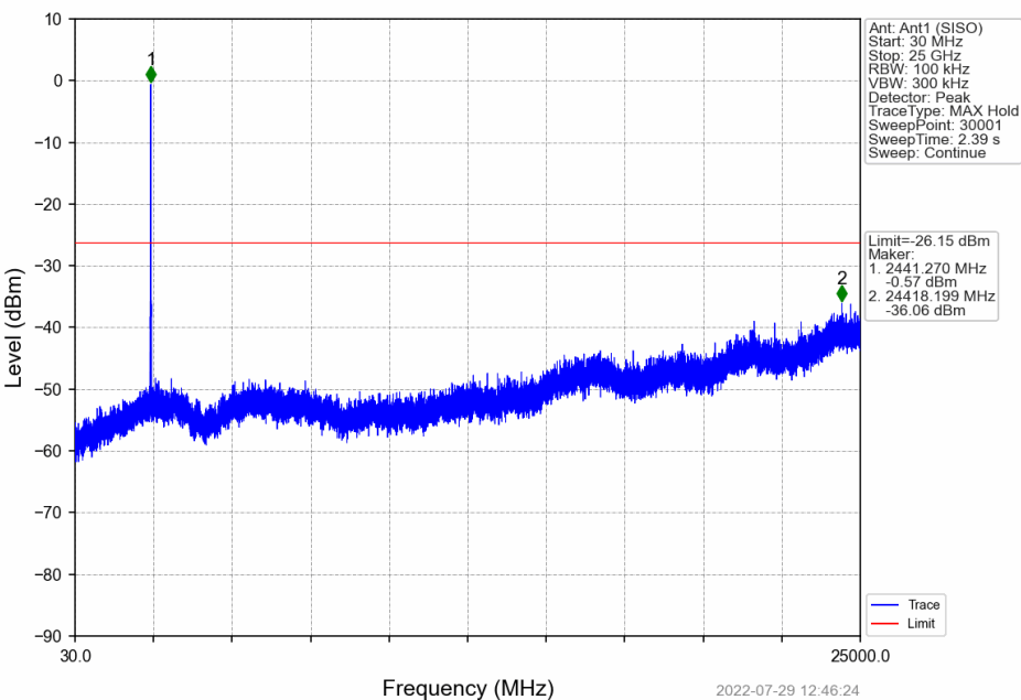
802.11g_MCH_2437MHz_Ant1 (SISO) NTN
