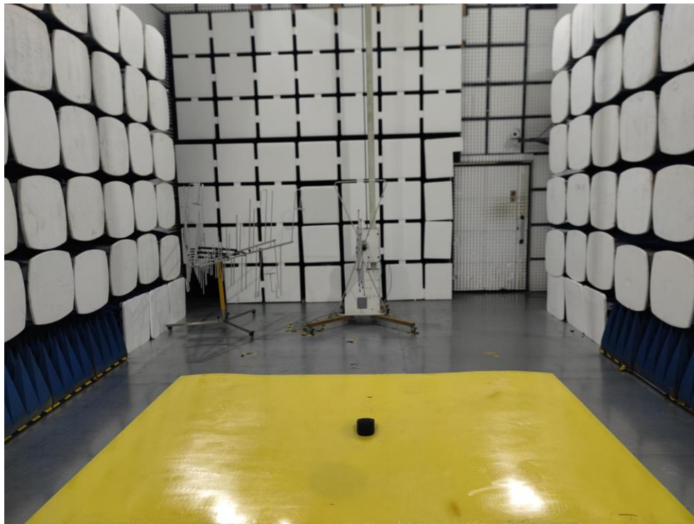
Fig. 1 (Below 1GHz)
