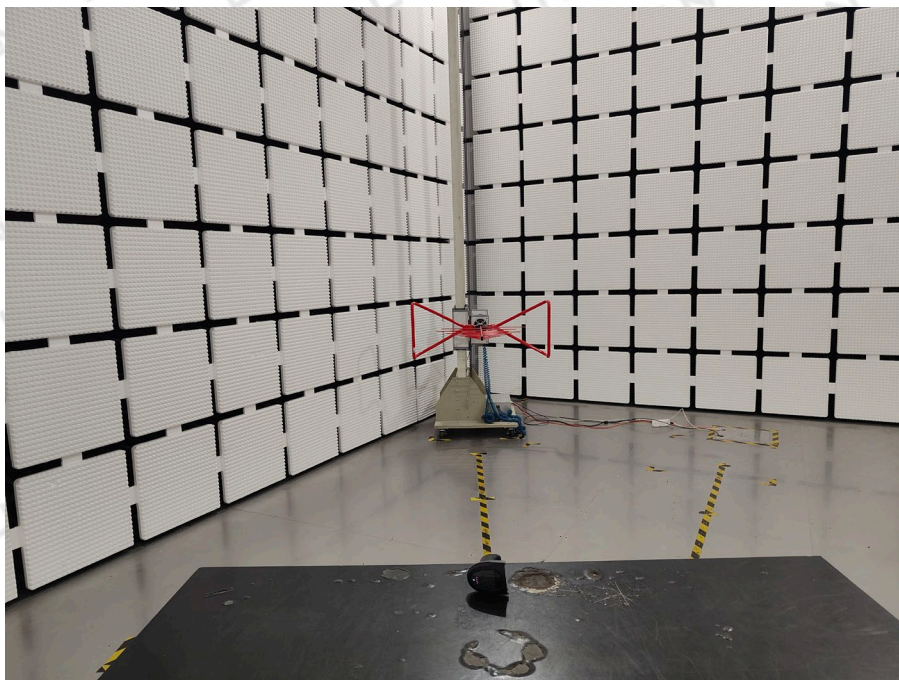
30MHz-1000MHz
