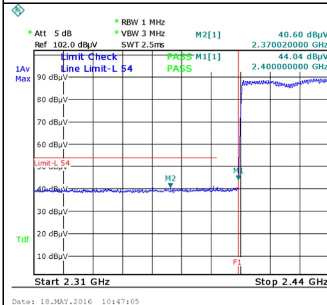
8DPSK--Hopping Left-AV
