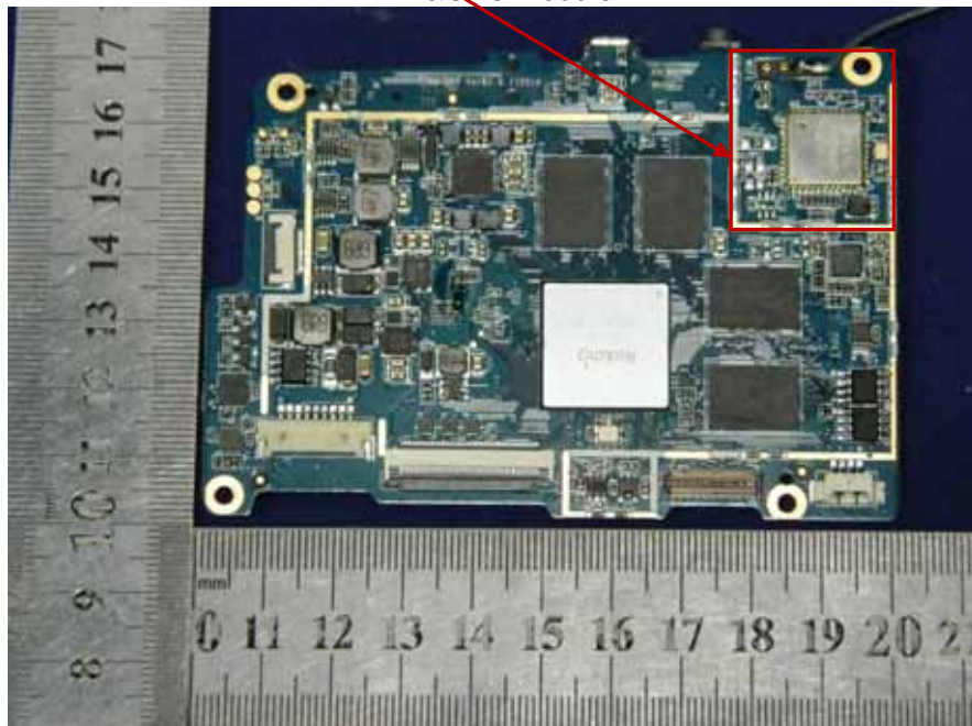
Wifi&GPS Module
