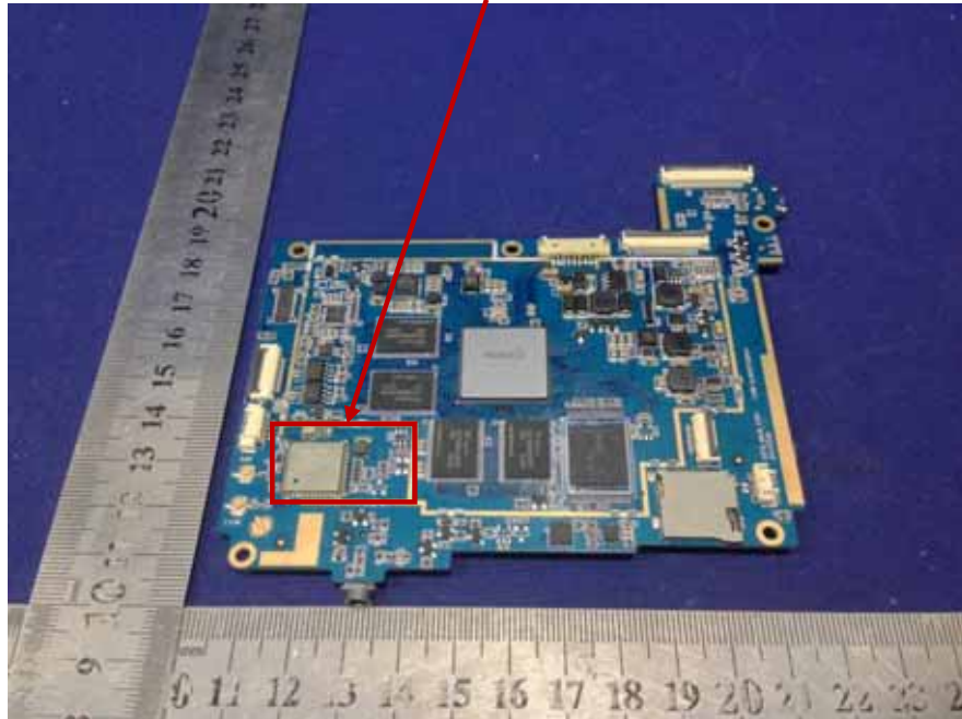
WIFI&BT&GPS Module
