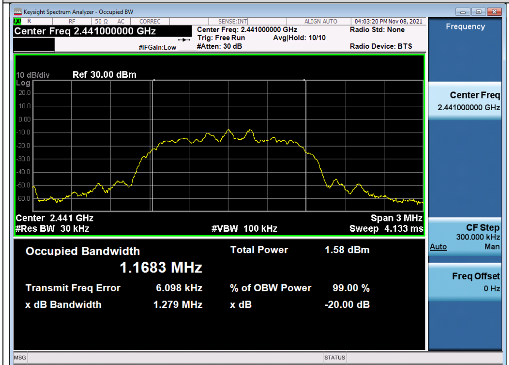
Test_Graph_EDR_ANT1_2441_2Mbps_OBW
