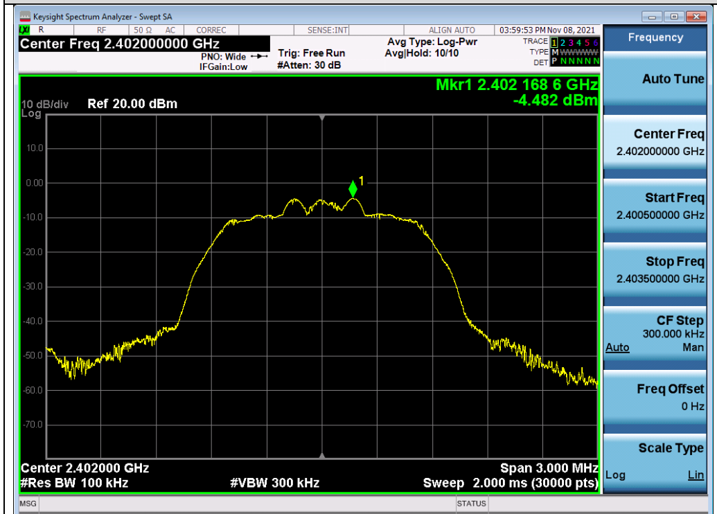
Test_Graph_EDR_ANT1_2402_2Mbps_Reference Level
