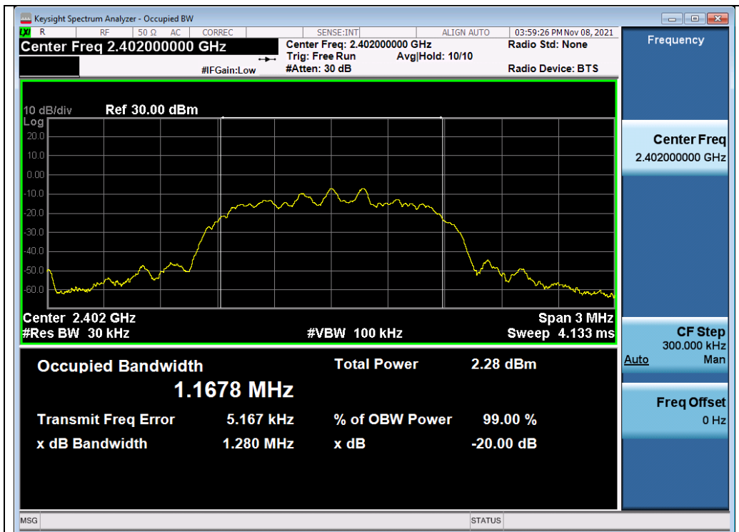
Test_Graph_EDR_ANT1_2402_2Mbps_OBW
