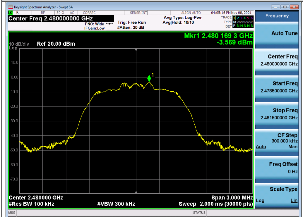
Test_Graph_EDR_ANT1_2480_2Mbps_Reference Level
