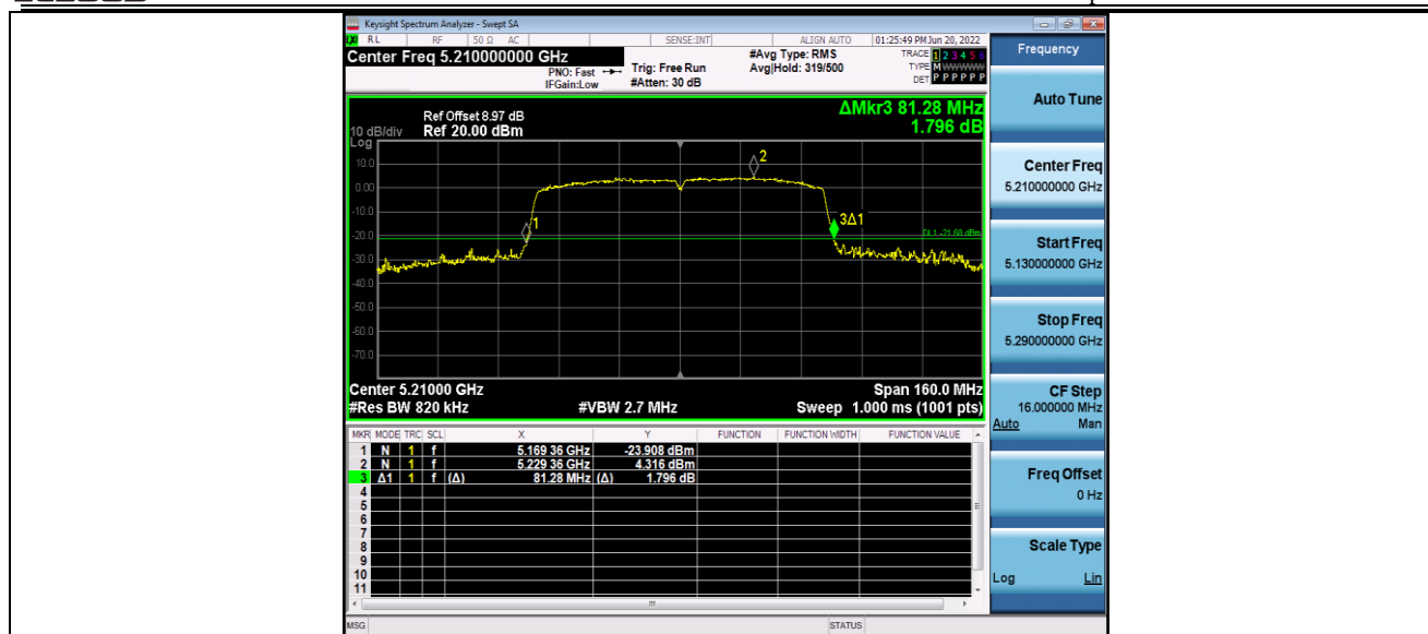
11AC80MIMO_Ant2_5210
