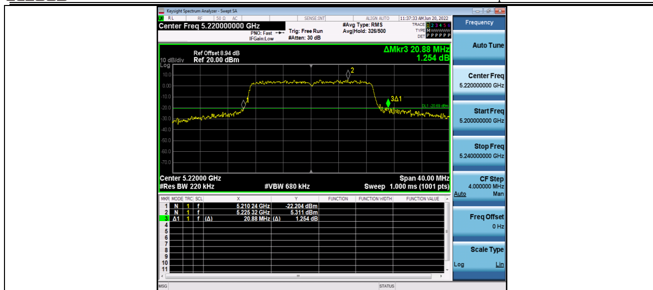
11AC20MIMO_Ant2_5220
