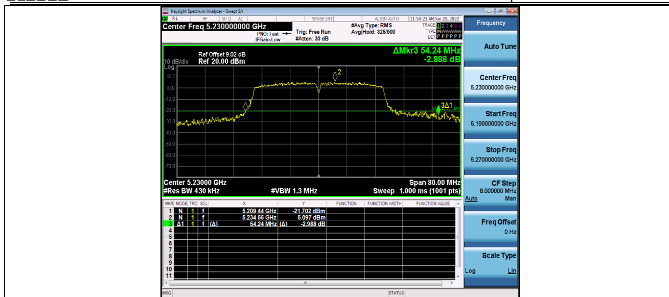
11AC40MIMO_Ant2_5230
