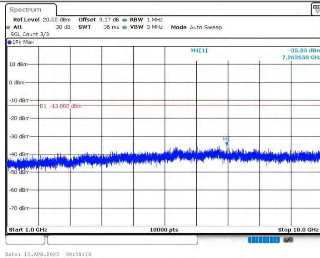
Band13-5MHz-QPSK-23255-1RB#0-Range2:1000~10000MHz
