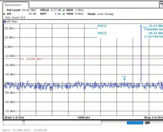
Band25-1.4MHz-QPSK-26047-1RB#0-Range2:1000~2000MHz
