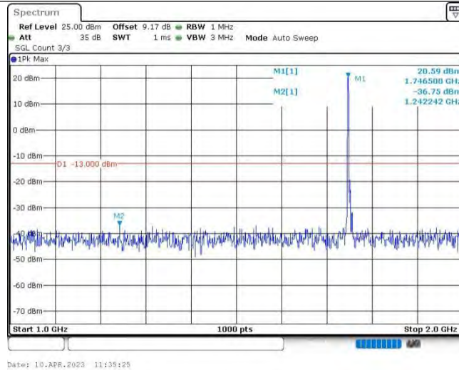
Band4-10MHz-QPSK-20350-1RB#0-Range2:1000~2000MHz
