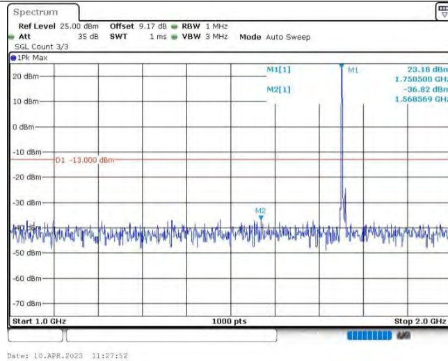
Band4-5MHz-QPSK-20375-1RB#0-Range2:1000~2000MHz
