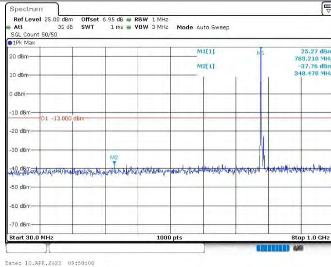
Band13-5MHz-QPSK-23255-1RB#0-Range1:30~1000MHz
