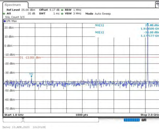
Band25-1.4MHz-QPSK-26683-1RB#0-Range2:1000~2000MHz
