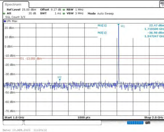
Band4-3MHz-16QAM-19965-1RB#0-Range2:1000~2000MHz
