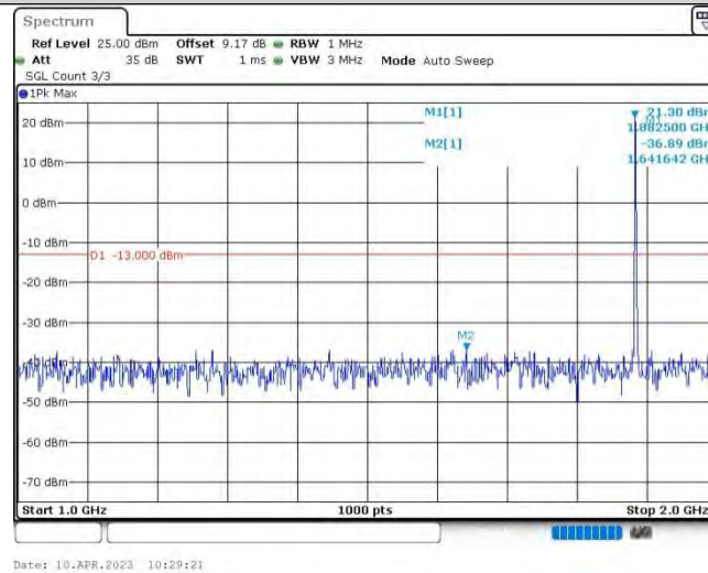
Band25-1.4MHz-QPSK-26365-1RB#0-Range2:1000~2000MHz
