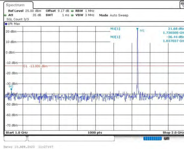
Band4-5MHz-QPSK-20175-1RB#0-Range2:1000~2000MHz
