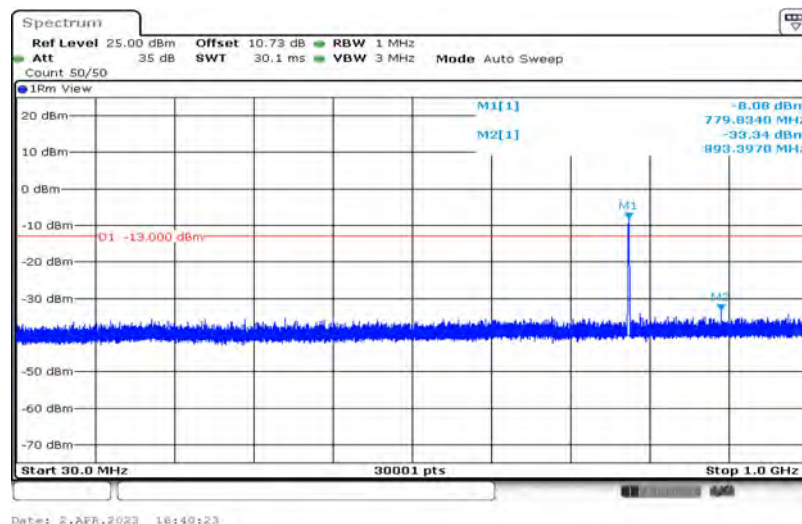
Band13-5MHz-QPSK-23230-1-0-Low-30-1000--33.34-PASS
