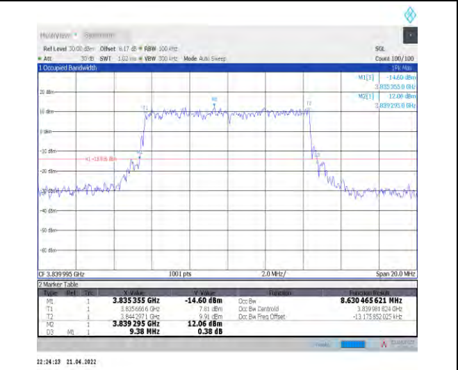
1-N77-3700-3980--30-10-M-3-DFT-16QAM-Outer_Fu ll-24@0-Ant0-8.63-9.380-≤10-PASS
