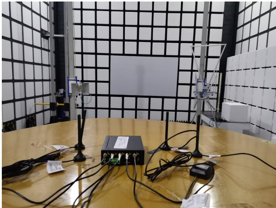
RSE
