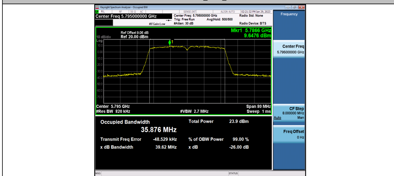
11AC40MIMO_Ant2_5795
