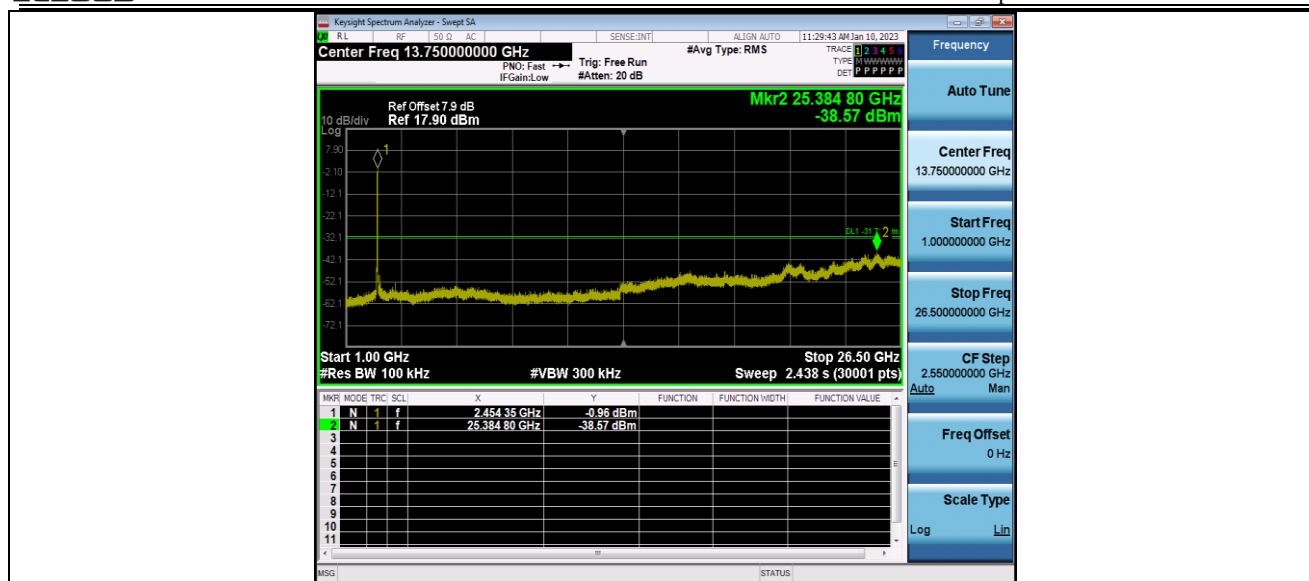
11N40MIMO_Ant2_2452_0~Reference
