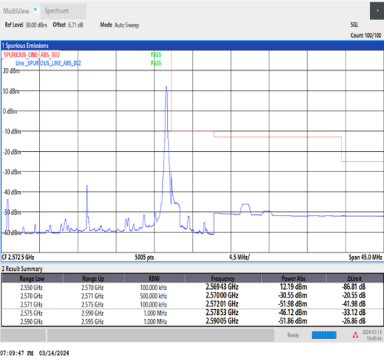
NTNV_CA_n7B_PC3_15+15_10+10_H+H_TID2_1_#1
