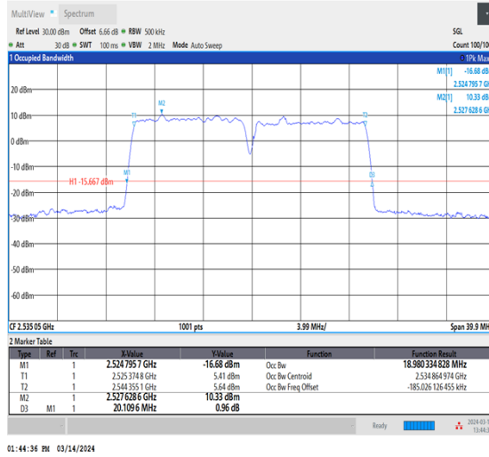
NTNV_CA_n7B_PC3_15+15_10+10_M+M_Ant1_TID8_1 _#1
