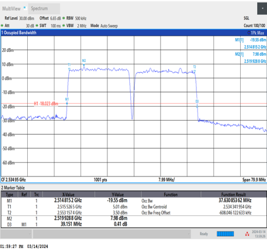
NTNV_CA_n7B_PC3_15+15_20+20_M+M_Ant1_TID6_1 _#1
