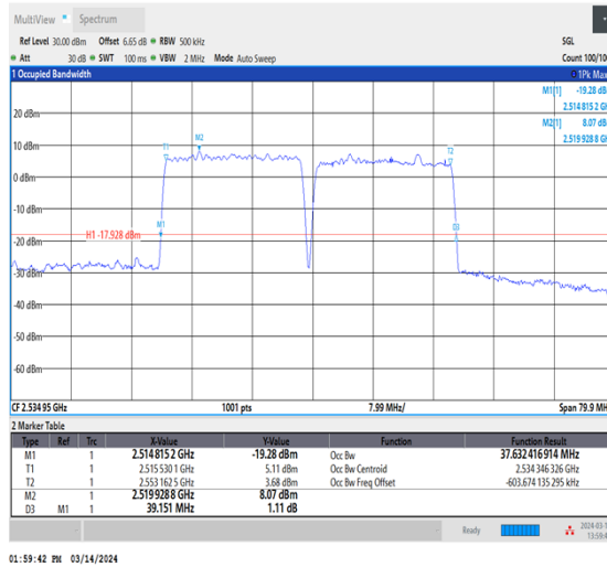
NTNV_CA_n7B_PC3_15+15_20+20_M+M_Ant1_TID7_1 _#1
