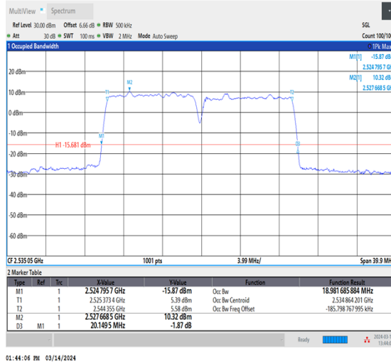
NTNV_CA_n7B_PC3_15+15_10+10_M+M_Ant1_TID6_1 _#1
