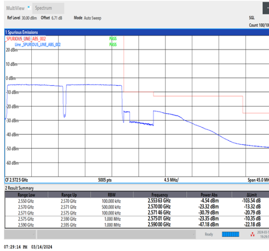
NTNV_CA_n7B_PC3_15+15_10+10_H+H_TID6_1_#1
