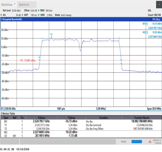
NTNV_CA_n7B_PC3_15+15_10+10_M+M_Ant1_TID7_1 _#1
