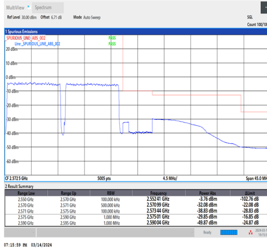
NTNV_CA_n7B_PC3_15+15_10+10_H+H_TID3_1_#1
