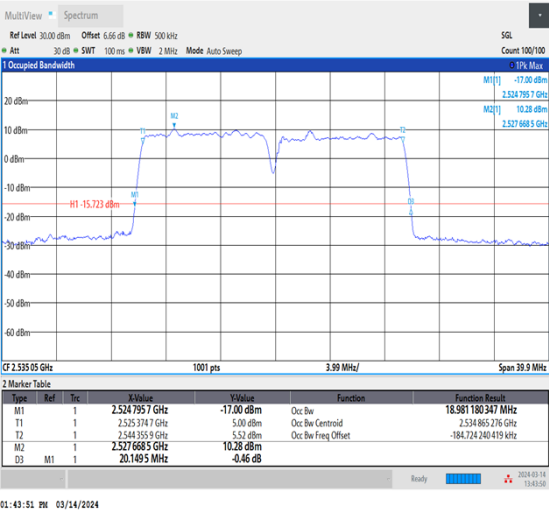
NTNV_CA_n7B_PC3_15+15_10+10_M+M_Ant1_TID5_1 _#1
