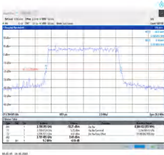
1-N78-3700-3800-30-10-L-7-CP-16QAM-Outer_Full-24@0-Ant0-8.584-9.200-≤10-PASS
