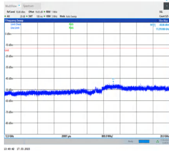
1-N71-PC3-15-20-L-1-DFT-PI2BPSK- Inner_1RB_Left-1@1-12000-20000-Ant7-17270.00-- 43.86--13-PASS
