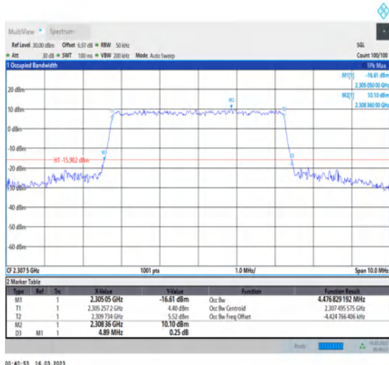
1-N30-PC3-15-5-L-7-CP-16QAM-Outer_Full-25@0-Ant1-4.477-4.890-≤5-PASS
