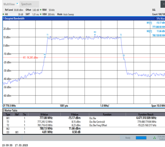
1-N13-PC3-15-5-L-1-DFT-QPSK-Outer_Full-25@0- Ant7-4.471-4.810-≤5-PASS
