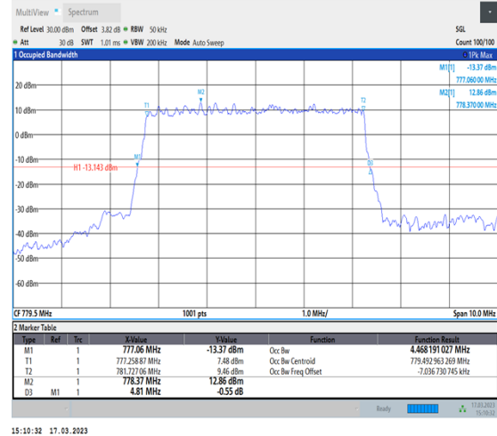
1-N13-PC3-15-5-L-2-DFT-PI2BPSK-Outer_Full- 25@0-Ant7-4.468-4.810-≤5-PASS
