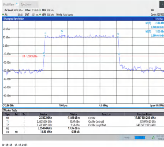
1-N7-PC3-15-20-H-2-DFT-PI2BPSK-Outet_Full-100@0-Ant1-17.867-18.520-≤20-PASS
