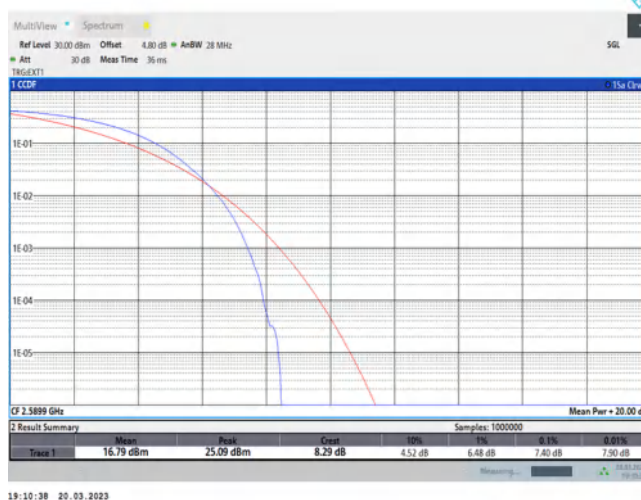
38-38-20MHz-20MHz-QPSK-QPSK-37901-38099-100RB#0-100RB#0
