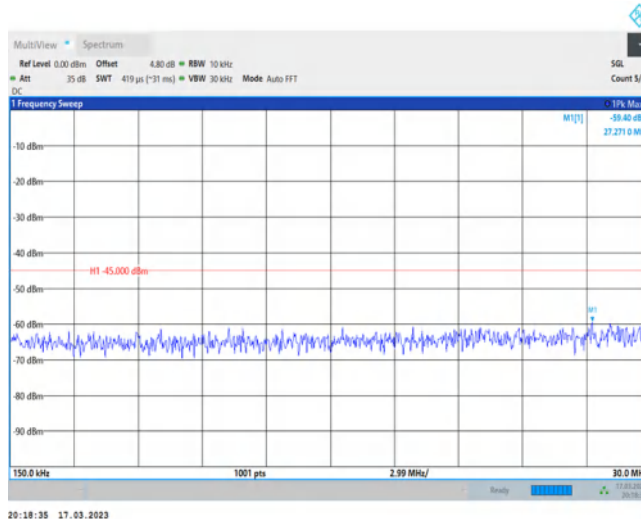
Band38-20MHz-QPSK-37850-1RB#0-Range2:0.15~30MHz
