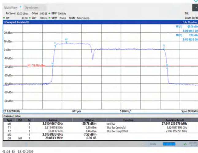
48-48-10MHz-20MHz-QPSK-QPSK-55896-56040-50RB#0-100RB#0
