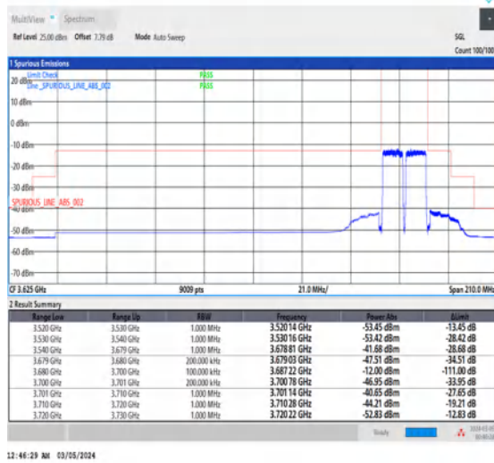
NTNV_CA_n48B_PC3_30+30_10+10_H+H_TID3_1_#1
