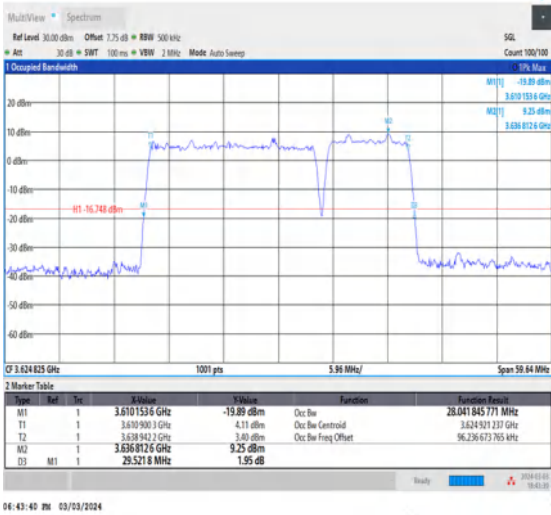
NTNV_CA_n48B_PC3_30+30_20+10_M+M_Ant0_TID8_1_#1
