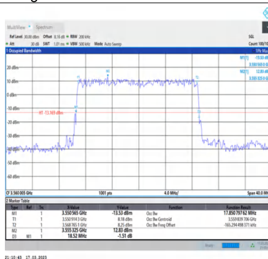
1-N48-PC3-30-20-L-2-DFT-PI2BPSK-Outer_Full-50@0-Ant0-17.851-18.520-≤20-PASS
