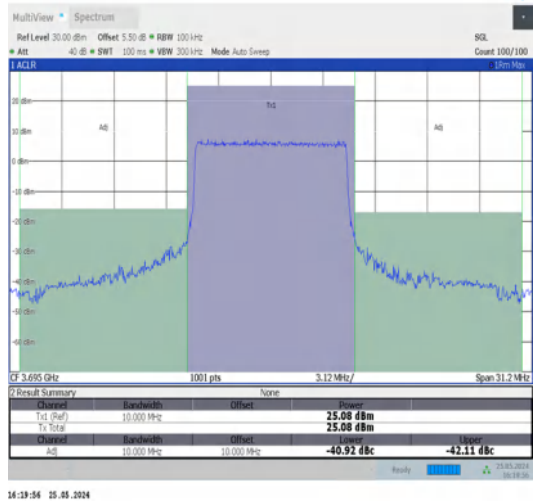
Band48-10MHz-QPSK-56690-50RB#0-PASS
