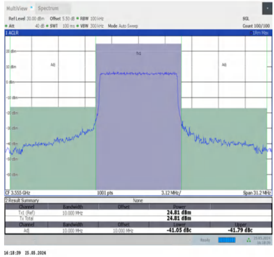
Band48-10MHz-QPSK-55290-50RB#0-PASS
