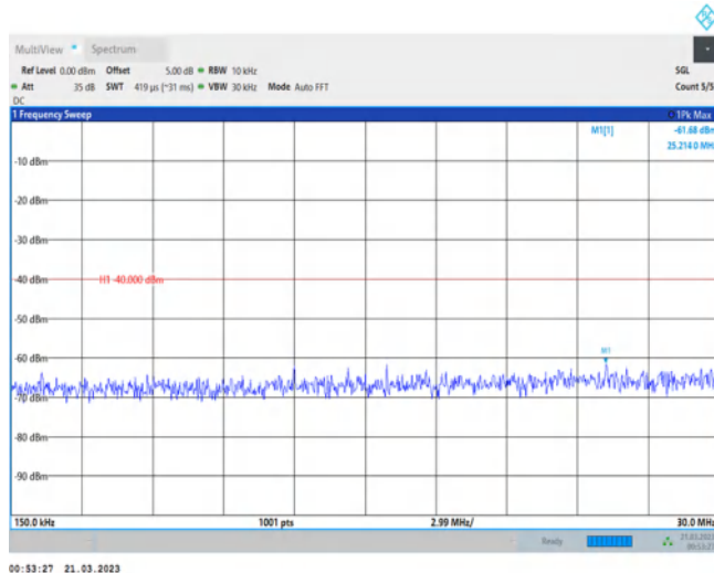
Band48-20MHz-QPSK-55340-1RB#0-Range2:0.15~30MHz
