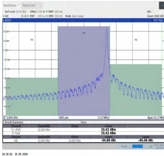
Band48-10MHz-QPSK-56690-1RB#49-PASS
