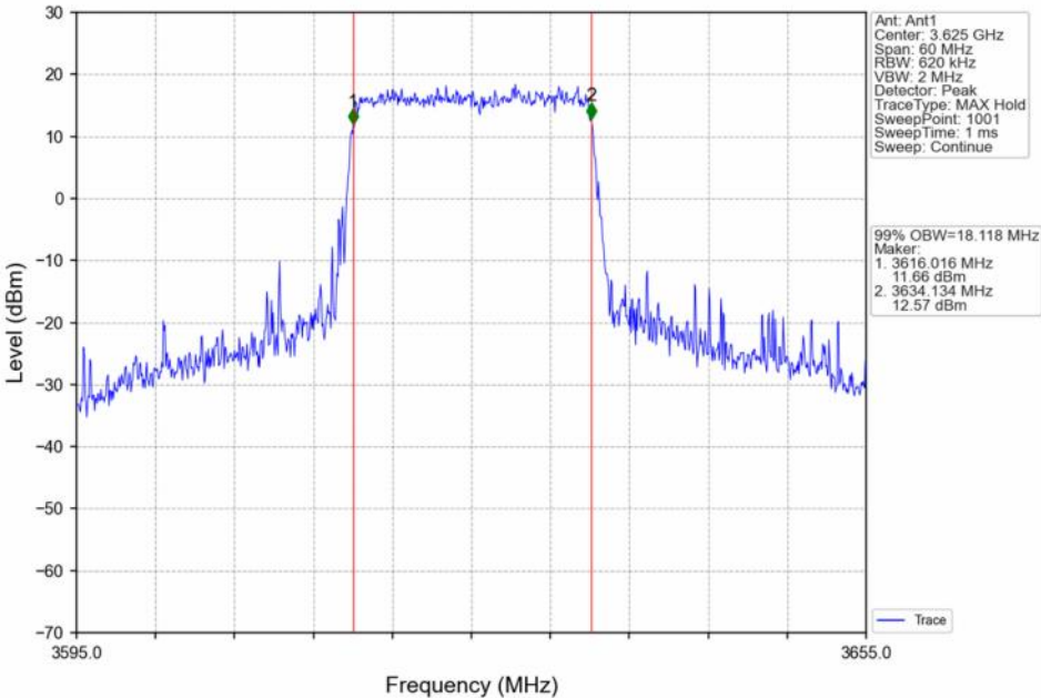
Band48_20MHz_QPSK_MCH_3625MHz_RB_100_0_NTNV
