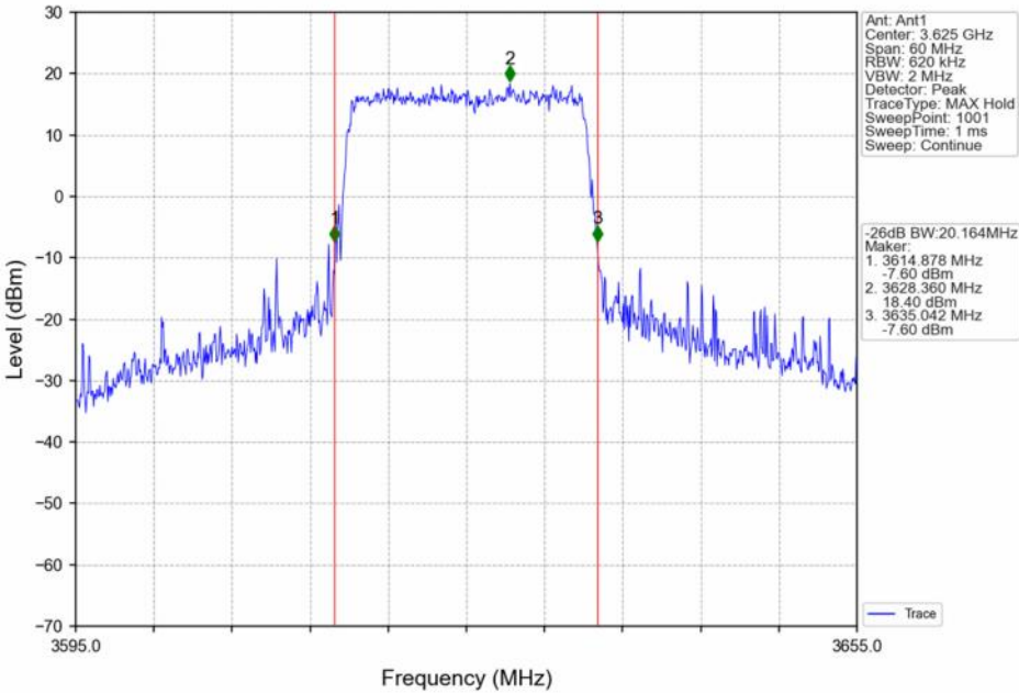
Band48_20MHz_QPSK_MCH_3625MHz_RB_100_0_NTNV
