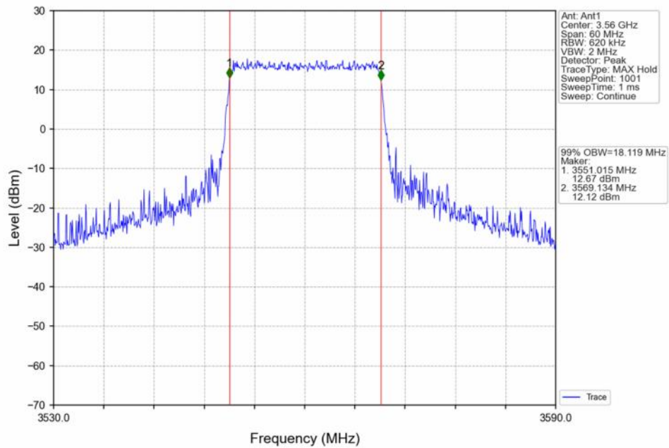
Band48_20MHz_16QAM_LCH_3560MHz_RB_100_0_NTNV
