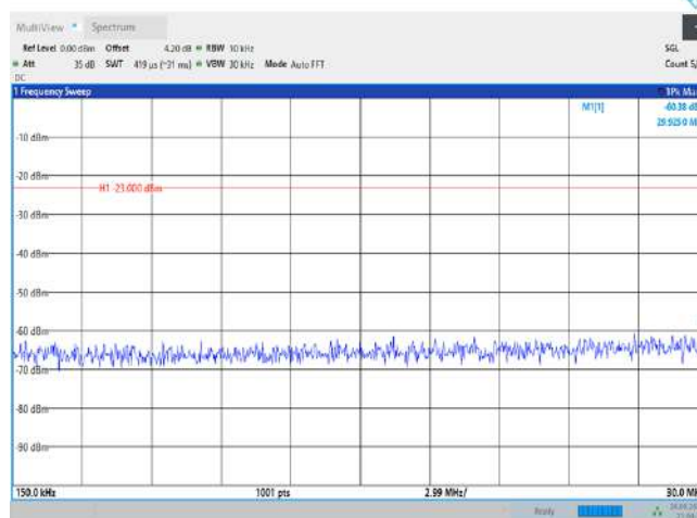
Band66-20MHz-QPSK-132072-1RB#0-Range2:0.15~30MHz
