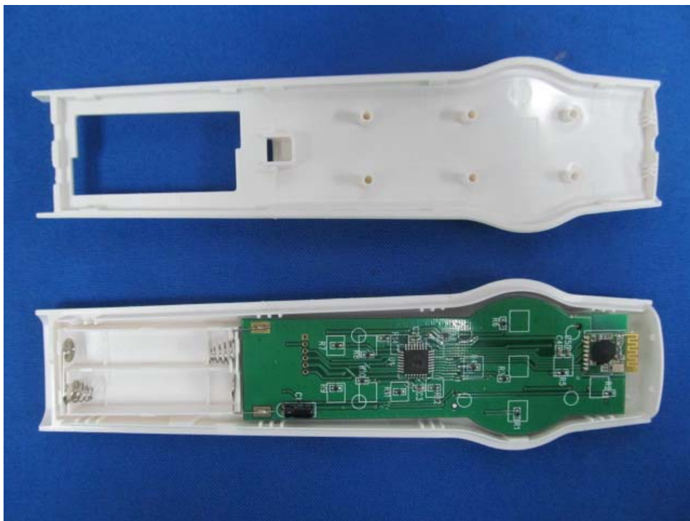
(2) EUT Photo
