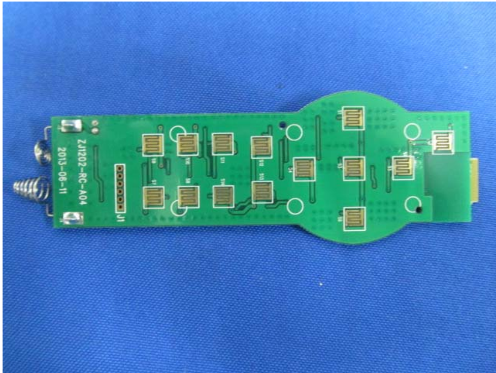
(4) EUT Photo
