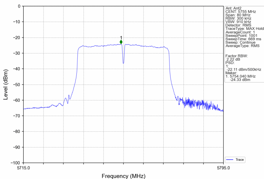
802.11n(HT40)_LCH_5755MHz_MIMO_NTNV
