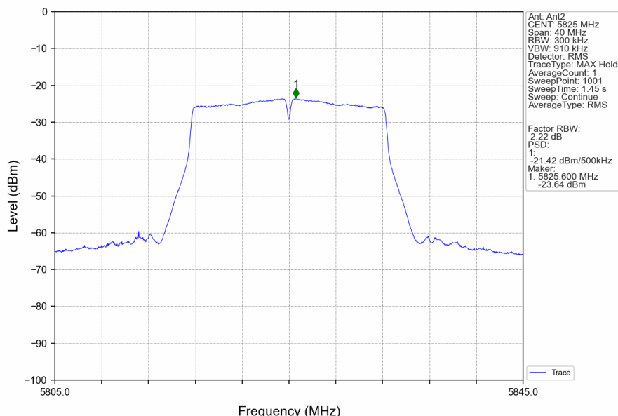
802.11a_HCH_5825MHz_Ant2_NTNV
