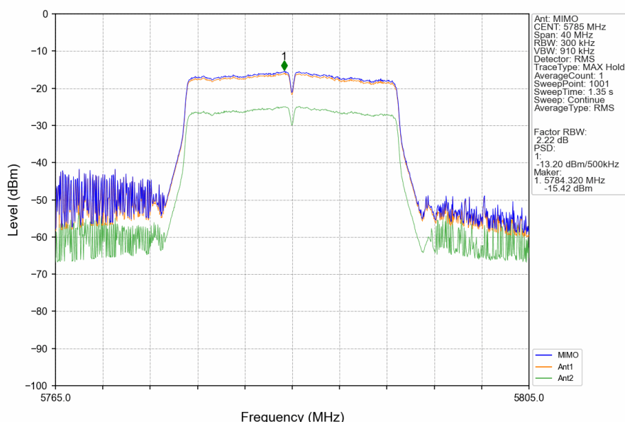
802.11n(HT20)_MCH_5785MHz_MIMO_NTNV
