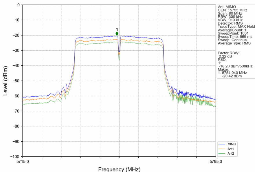
802.11n(HT40)_LCH_5755MHz_MIMO_NTNV
