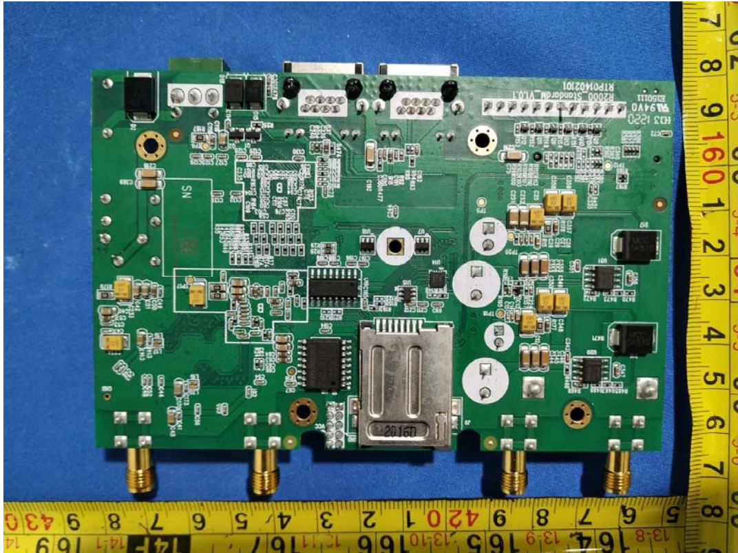
WWAN Module
