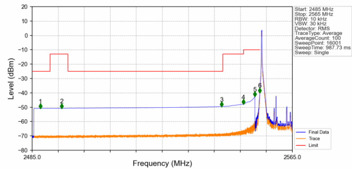
Band41_10MHz_QPSK_LCH_2560MHz_RB_1_0_NTNV
