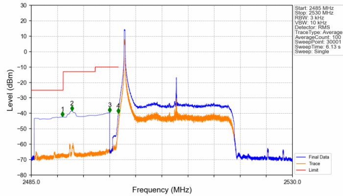
Band7_20MHz_QPSK_LCH_2510MHz_RB_1_0_NTNV
