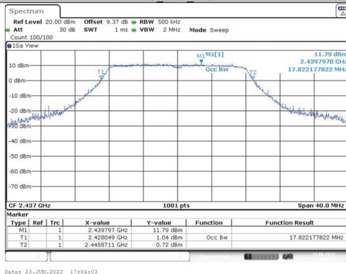
11G_Ant2_2437
