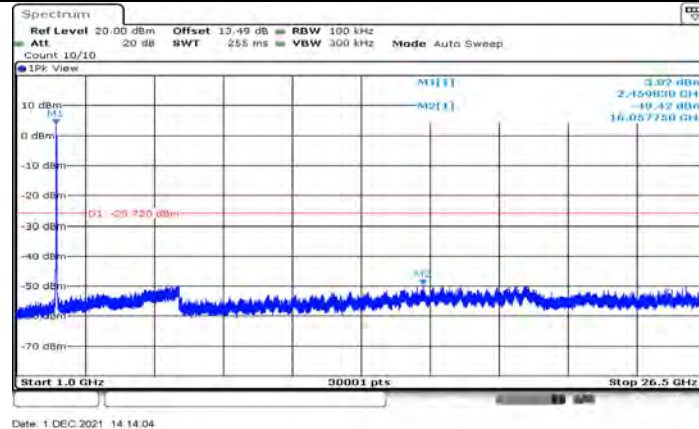
11N20MIMO Ant2 2462 1000-26500
