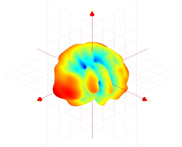
3D方向图
