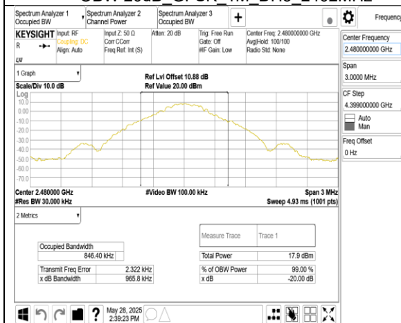
OBW 20dB GFSK 1M DH5 2480MHz
