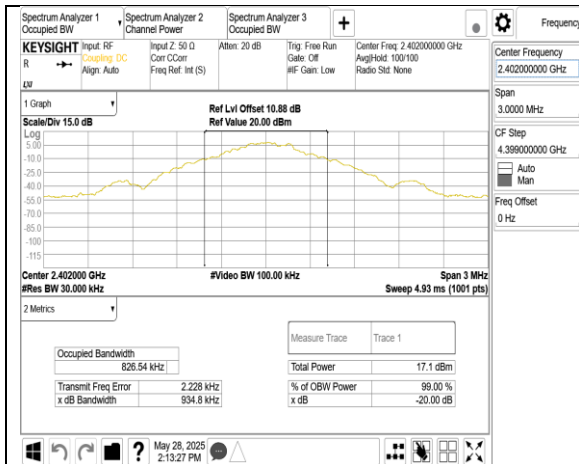
OBW 20dB GFSK 1M DH5 2402MHz
