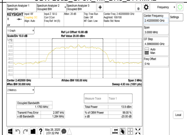
OBW 20dB \pi/4 DQPSK 2M DH5 2402MHz
