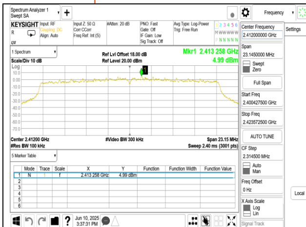
802.11ax_20MHz_Chain0_2412MHz
