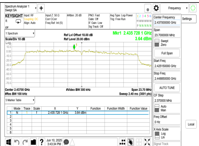
802.11ax_20MHz_Chain0_2437MHz
