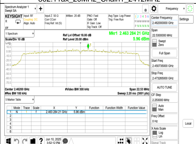
802.11ax_20MHz_Chain1_2462MHz
