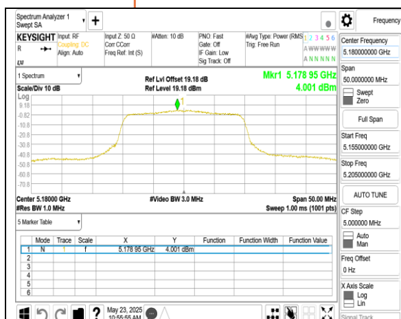
802.11ax_20MHz_Chain0_5180MHz
