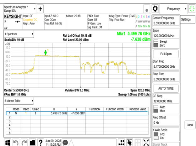
802.11ax_80MHz_Chain0_5530MHz_RU484_65
