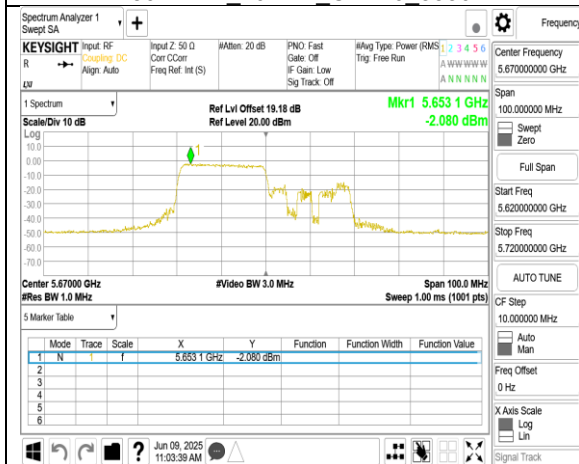
802.11ax 40MHz Chain0 5670MHz RU242_62
