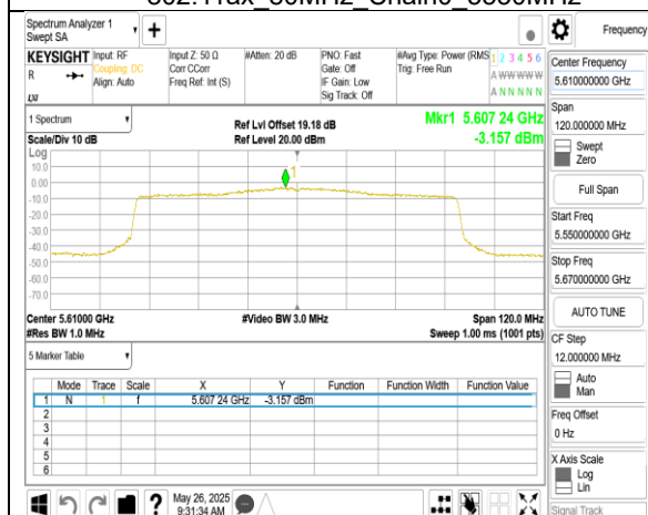
802.11ax_80MHz_Chain0_5610MHz
