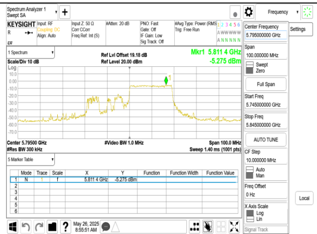
802.11ax 40MHz Chain1 5795MHz RU242 62
