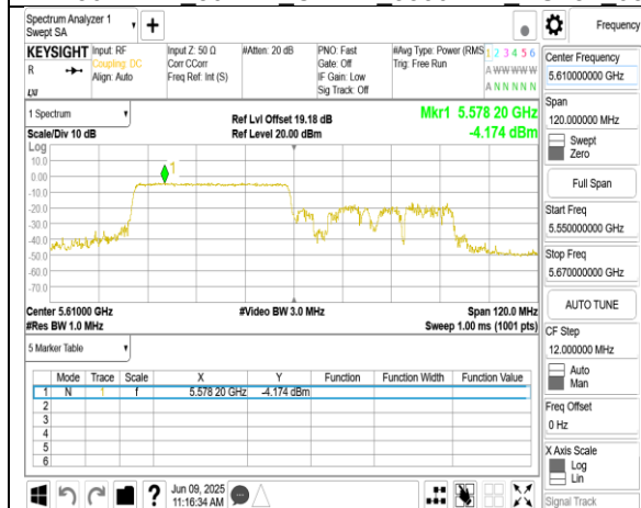
802.11ax 80MHz Chain1 5610MHz RU484 66
