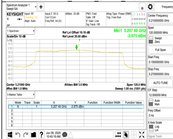
802.11ax 80MHz Chain0 5210MHz
