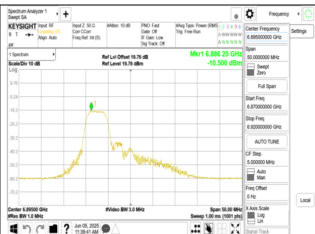
802.11ax 20MHz Chain1 6895MHz RU52_37
