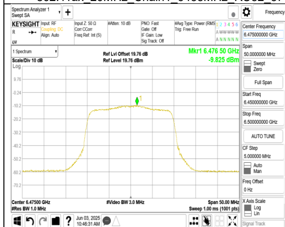
802.11ax 20MHz Chain1 6475MHz
