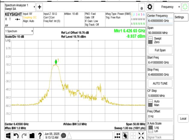
802.11ax_20MHz_Chain1_6435MHz_RU26_0
