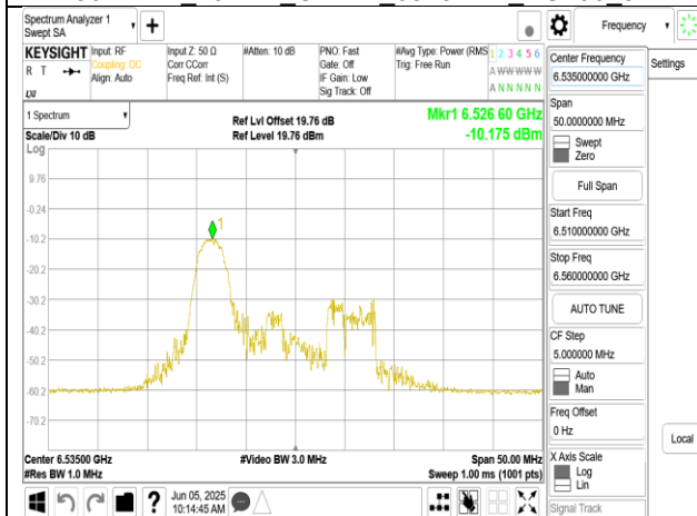
802.11ax 20MHz Chain1 6535MHz RU26_0
