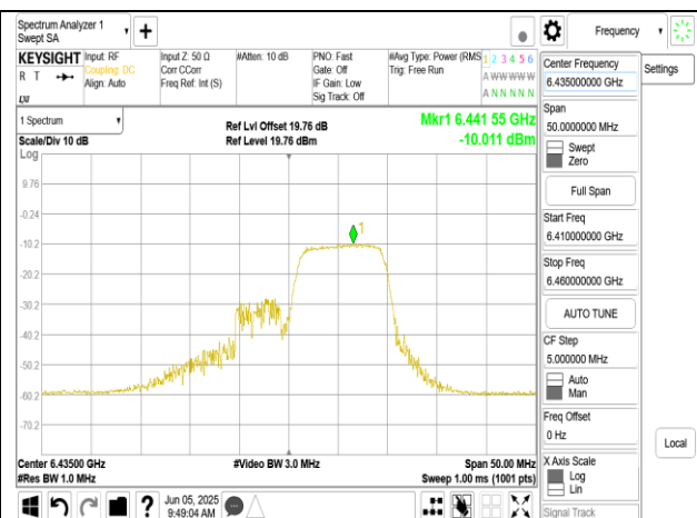
802.11ax 20MHz Chain1 6435MHz RU106 53
