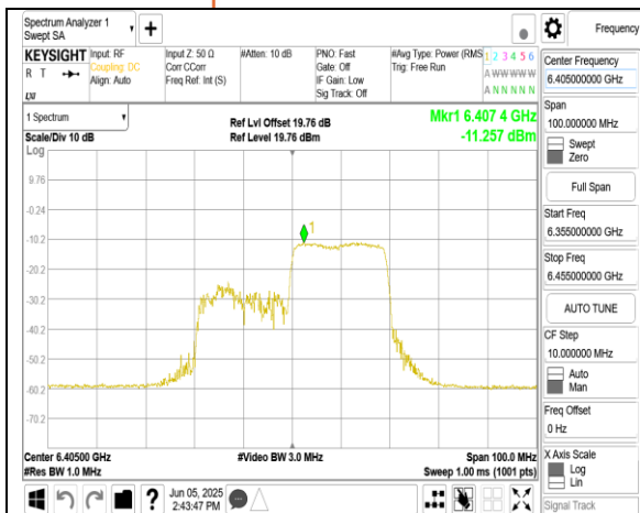
802.11ax 40MHz Chain0 6405MHz RU242_62
