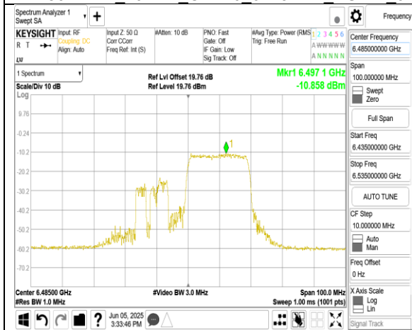
802.11ax 40MHz Chain0 6485MHz RU242_62
