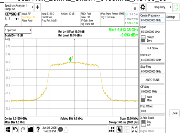
802.11ax 20MHz Chain1 6515MHz
