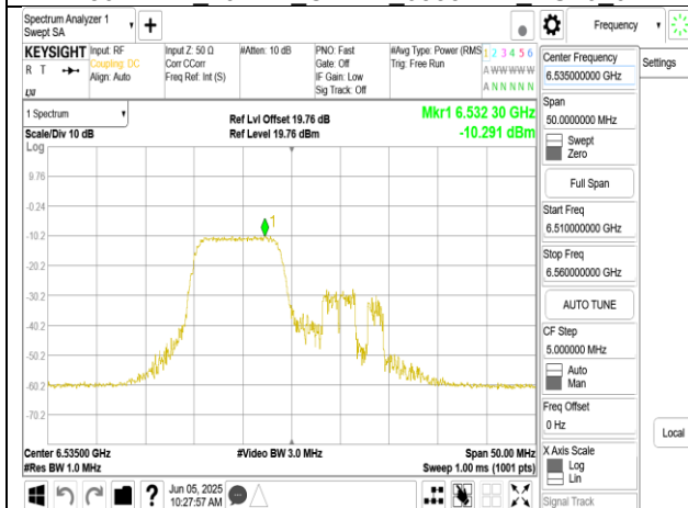
802.11ax 20MHz Chain1 6535MHz RU106_53
