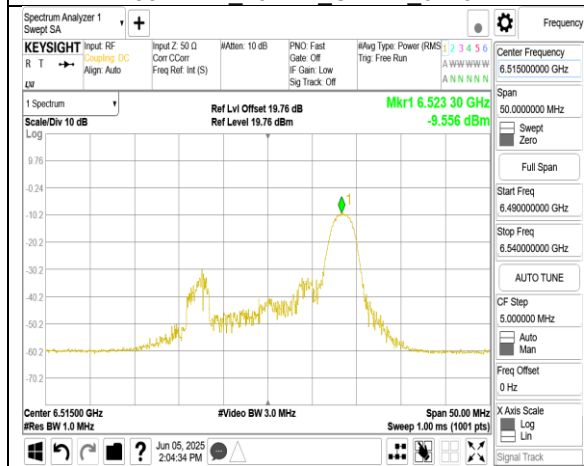
802.11ax 20MHz Chain1 6515MHz RU26 8
