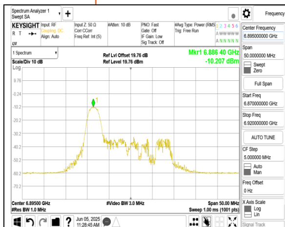
802.11ax 20MHz Chain1 6895MHz RU26_0
