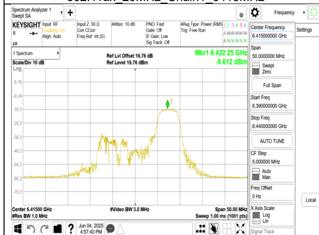
802.11ax_20MHz_Chain1_6415MHz_RU52_40
