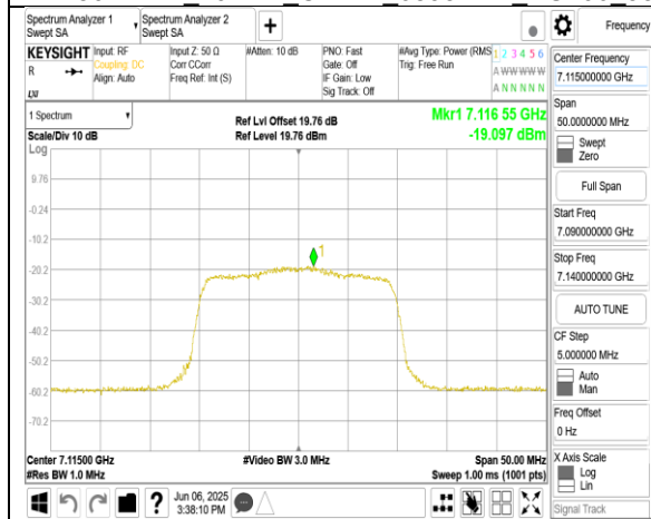
802.11ax 20MHz Chain1 7115MHz
