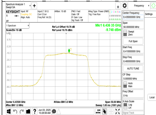
802.11ax_20MHz_Chain1_6435MHz
