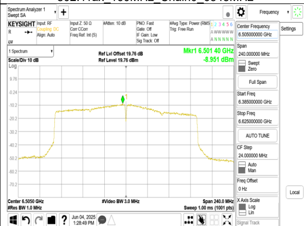
802.11ax_160MHz_Chain0_6505MHz
