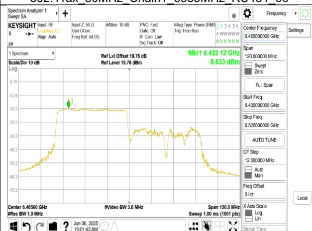
802.11ax_80MHz_Chain1_6465MHz_RU484_65
