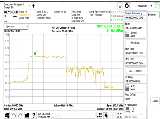
802.11ax_160MHz_Chain0_6665MHz_RU996_67
