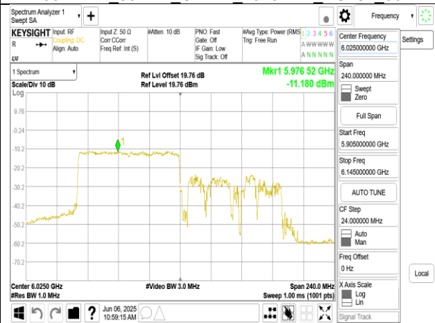
802.11ax 160MHz Chain0 6025MHz RU996 67
