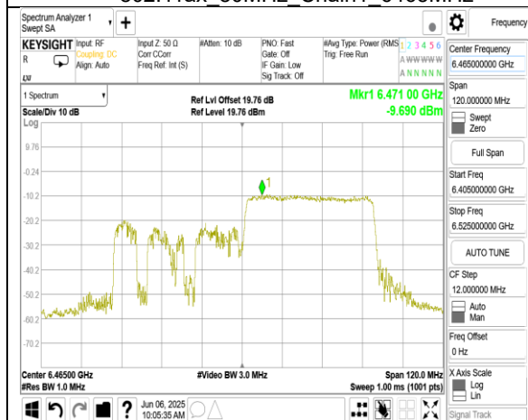
802.11ax_80MHz_Chain1_6465MHz_RU484_66
