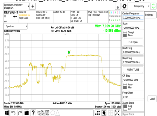
802.11ax 80MHz Chain1 7025MHz RU484 66
