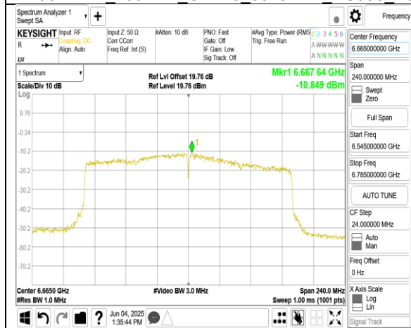
802.11ax_160MHz_Chain0_6665MHz
