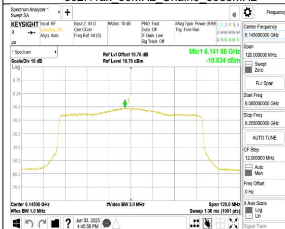
802.11ax 80MHz Chain0 6145MHz
