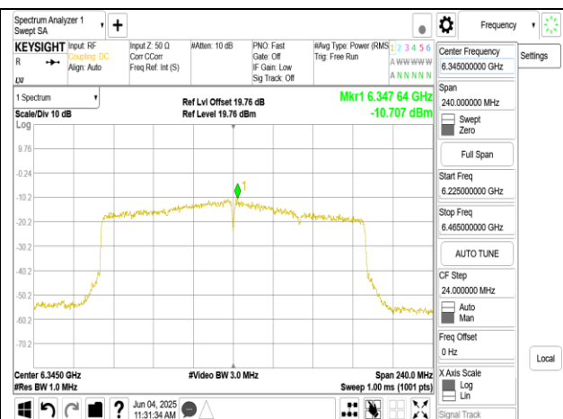
802.11ax_160MHz_Chain0_6345MHz
