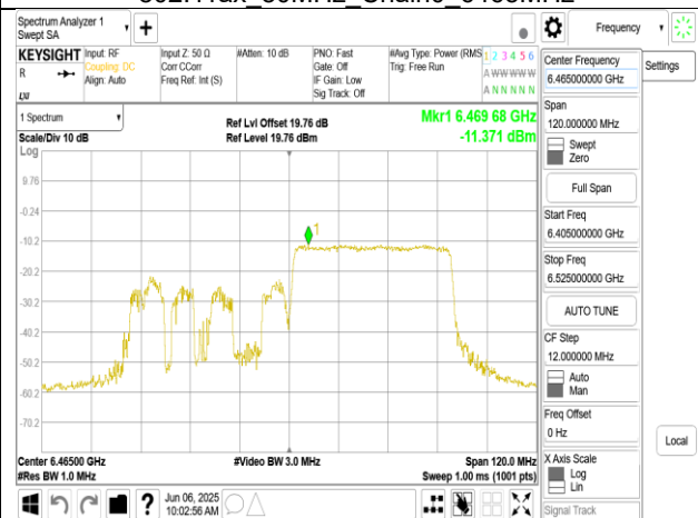
802.11ax 80MHz Chain0 6465MHz RU484 66
