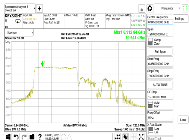
802.11ax 80MHz Chain1 6945MHz RU484 65
