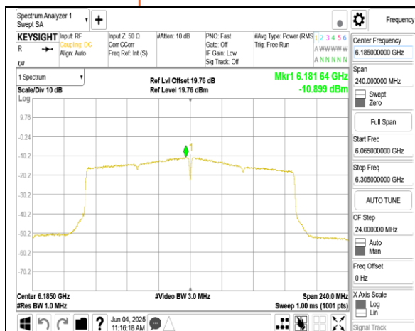
802.11ax_160MHz_Chain0_6185MHz
