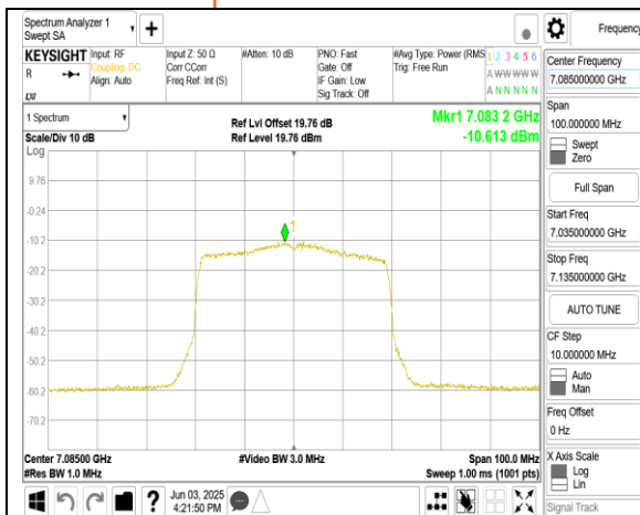
802.11ax 40MHz Chain1 7085MHz
