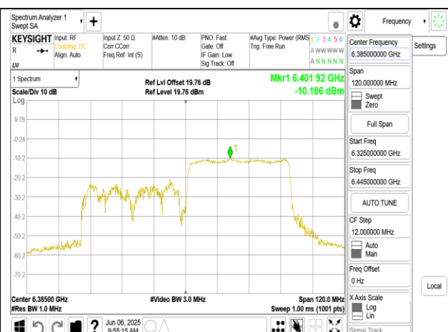
802.11ax_80MHz_Chain1_6385MHz_RU484_66
