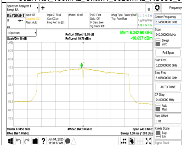
802.11ax 160MHz Chain1 6345MHz
