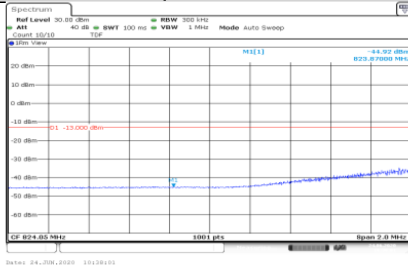
5-5-MHz-10MHz-QPSK-20428-20500-25RB#0-50RB#0
