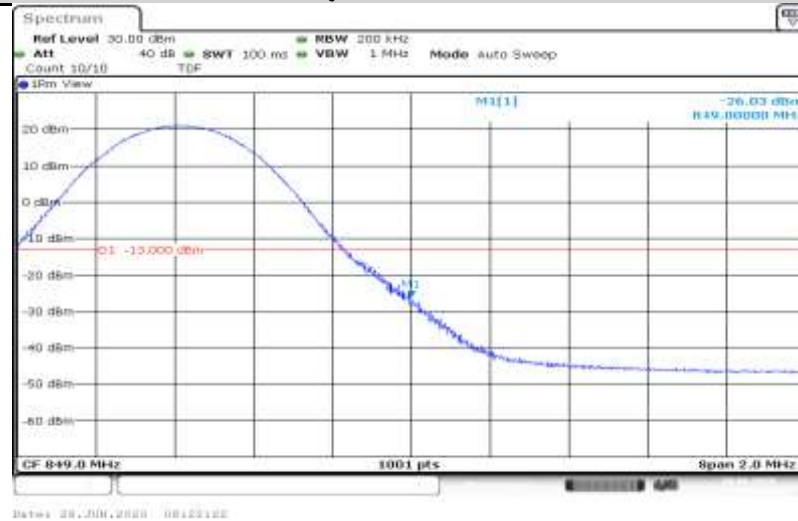
5-5-10MHz-10MHz-QPSK-20501-20600-50RB#0-50RB#0
