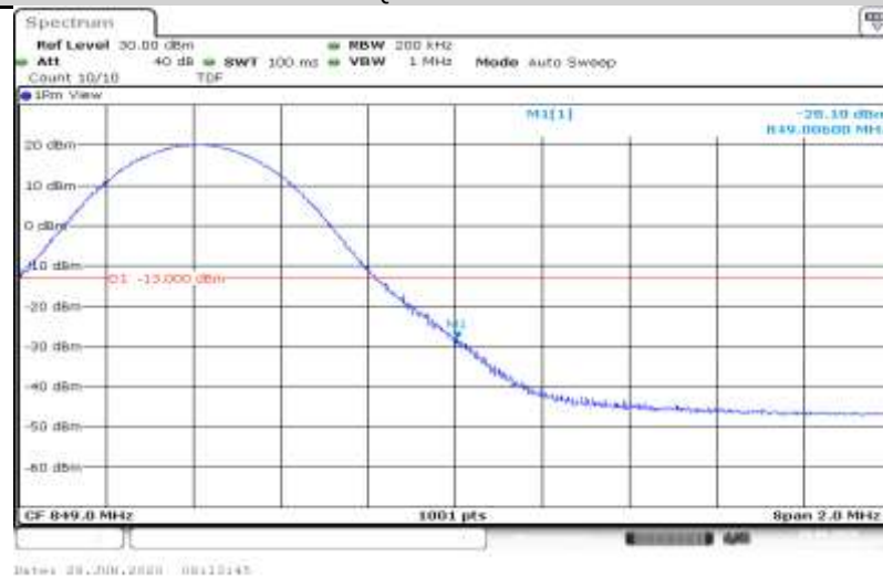
5-5-10MHz-10MHz-16QA M-20501-20600-50RB#0-50RB#0
