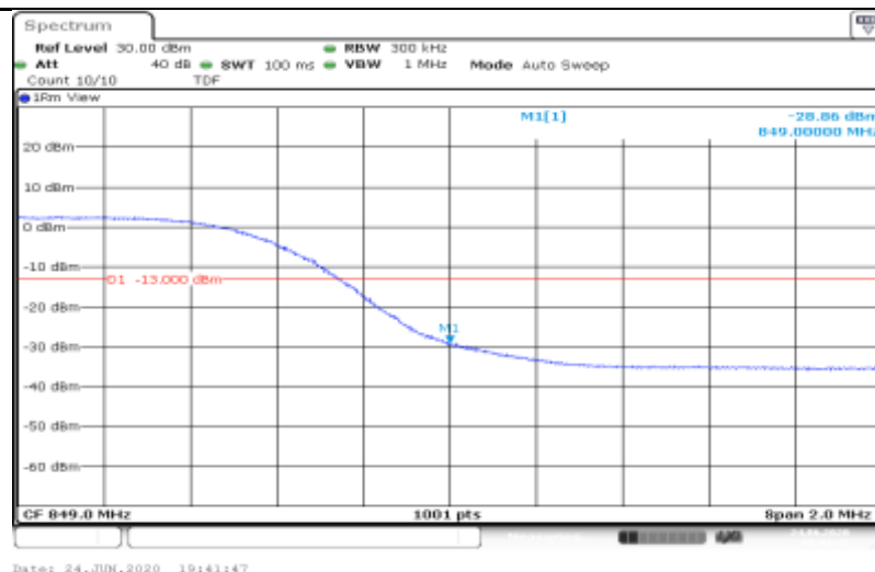
5-5-5MHz-10MHz-16QA M-20428-20500-1RB#0-0RB#0
