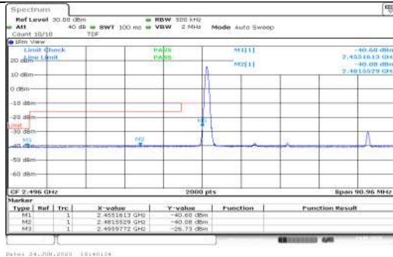
41-41-20MHz-20MHz-QPSK-41292-41490-0RB#0-1RB#99
