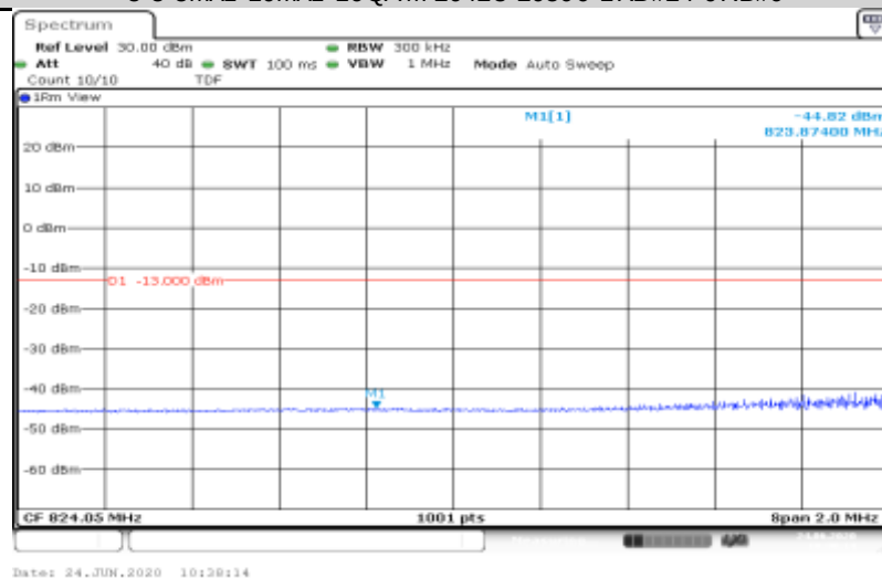
5-5-5MHz-10MHz-16QA M-20428-20500-25RB#0-50RB#0
