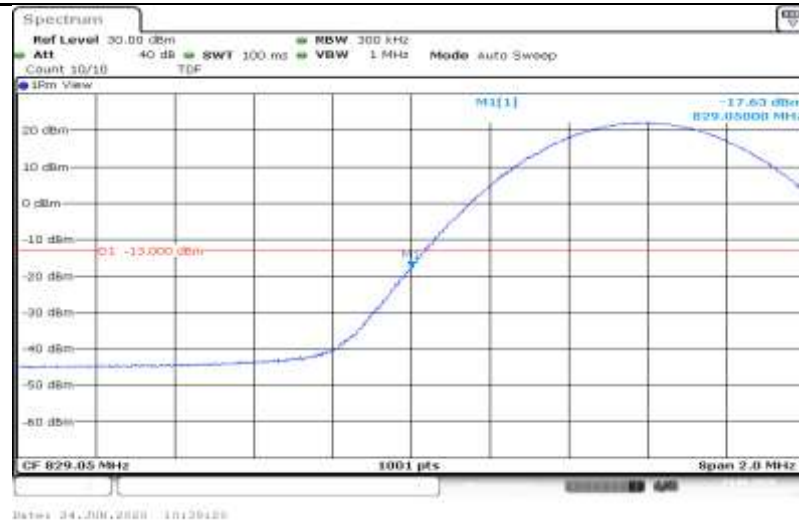
5-5MHz-10MHz-QPSK-20478-20550-1RB#24-0RB#0
