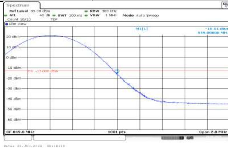
5-5MHz-10MHz-QPSK-20528-20600-25RB#0-50RB#0
