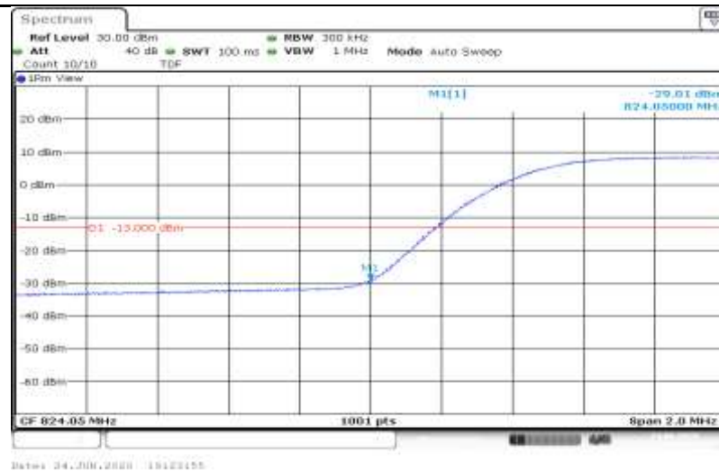
5-5-5MHz-10MHz-16QA M-20478-20550-1RB#0-0RB#0
